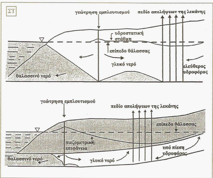
Σχήμα 2. Μέθοδοι αντιμετώπισης θαλάσσιας διείσδυσης (Πηγή: Πεταλάς κ.ά. 2002).
