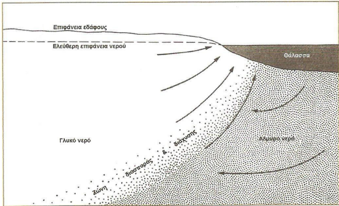
Σχήμα 1. Θαλάσσια διείσδυση σε ελεύθερο υδροφόρα.
